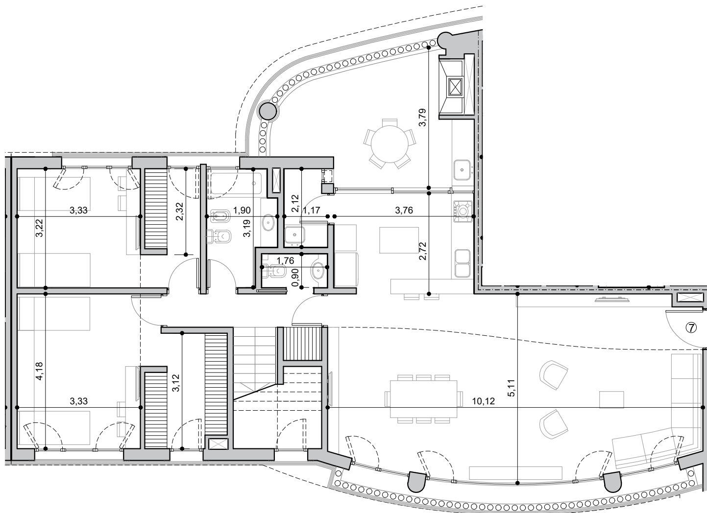
Duplex Ingreso y Dormitorios Nivel 2
